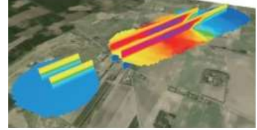
TEM 비저항 심도별 3D slices
