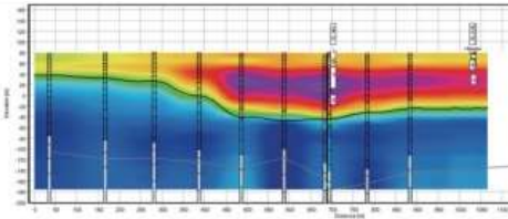
TEM 비저항 프로파일
