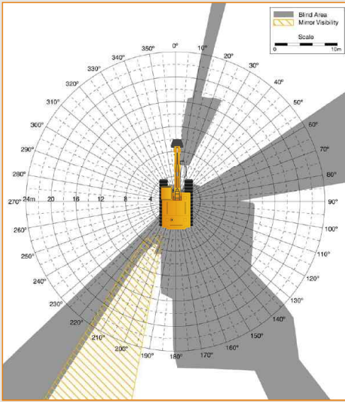
굴삭기 음영구역 (Blind Spots)
