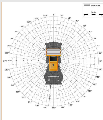
지게차, 로더, 롤러 등 주행장비 음영구역 (Blind Spots)
