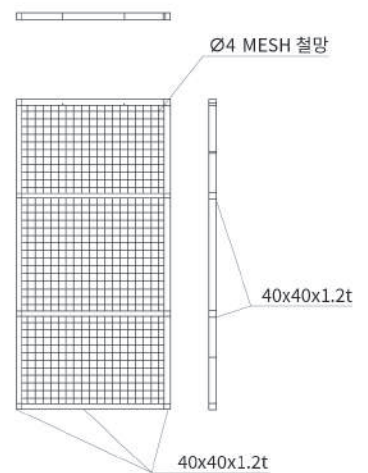
후면(Rear View)
